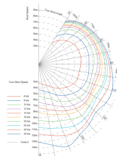
Polar Diagram Polaire de vitesse Deep draft and Classic rig
